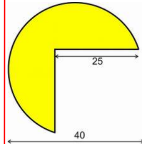
Eckschutz Typ A
